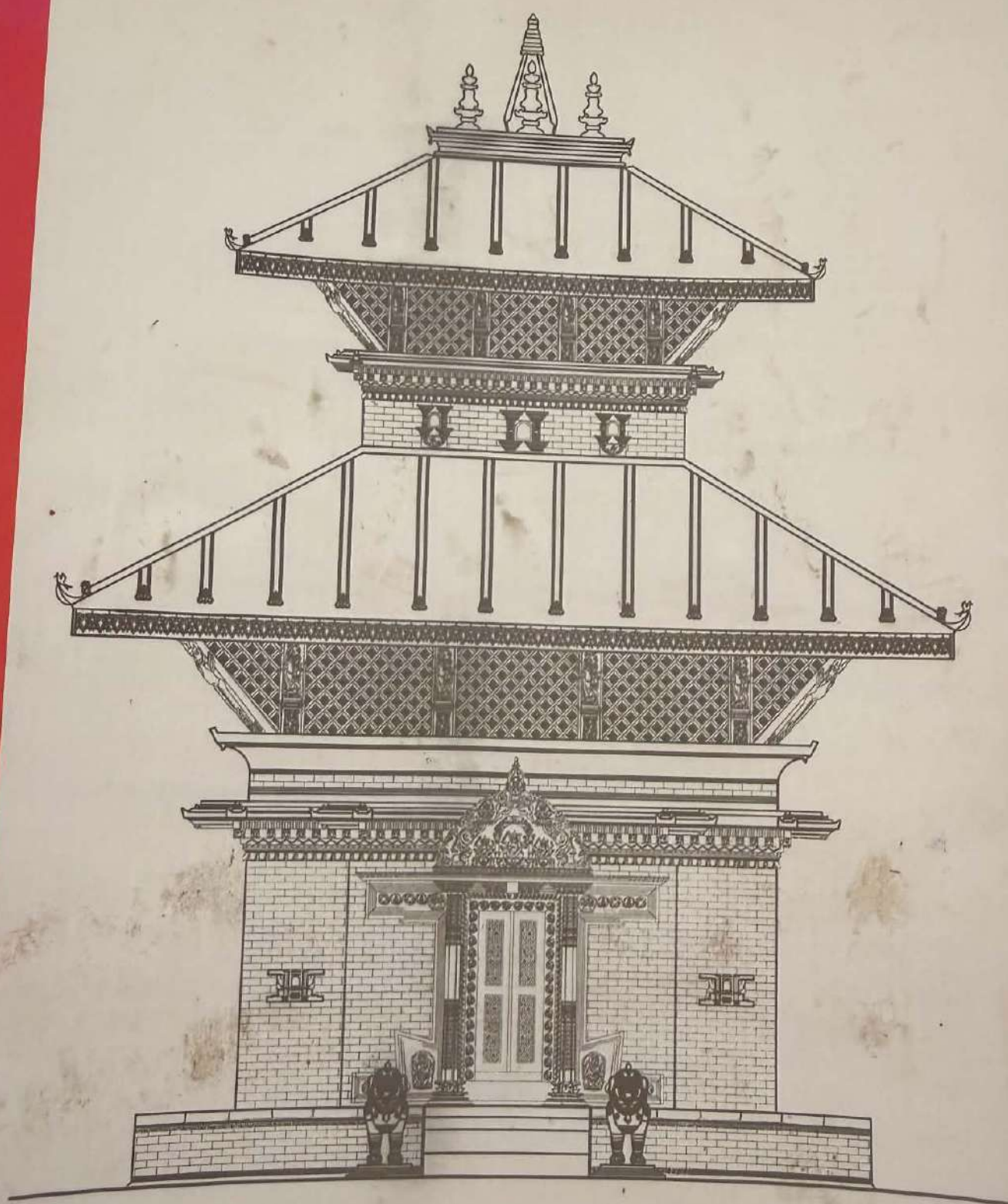
निर्माणाधिन भैरव मन्दिरको नक्सा
